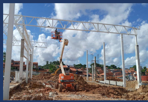
Montagem da estrutura metálica
